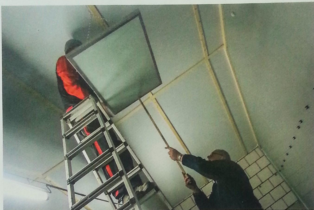
Kees van Roekel installeert de lichtplaten. Vijf platen van 1,20 x 60 centimeter verwarmen de speenbiggenafdeling van 120 vierkante meter met 220 biggen. FOTO'S: MATTHIJS VERHAGEN
